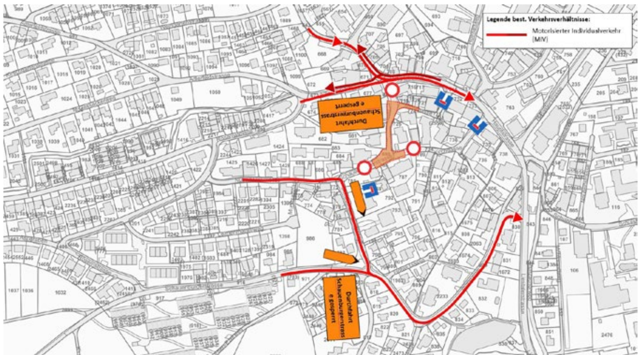
Bauphase 7 (Umleitung MIV Schauenburgerstrasse)
