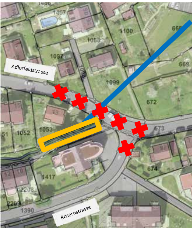
Einlaufbauwerk (orange), Bypass (blau), Sperrung (rot)
